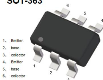
SOT-363
